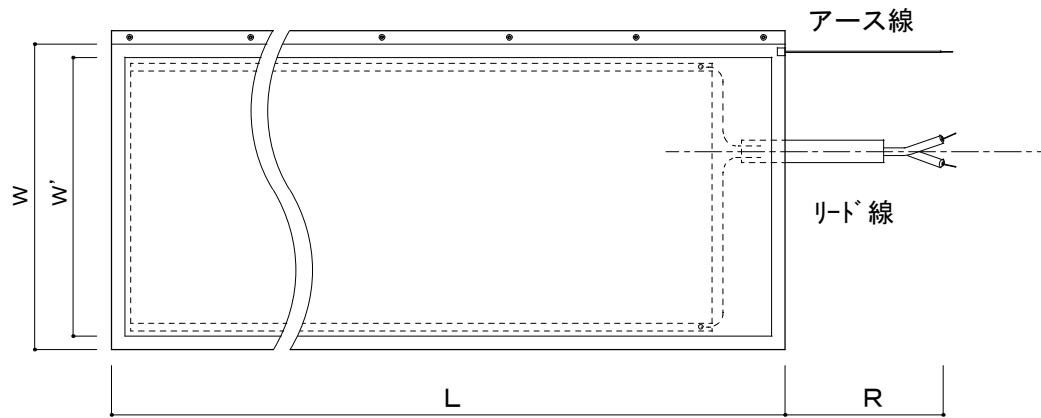
平面図
