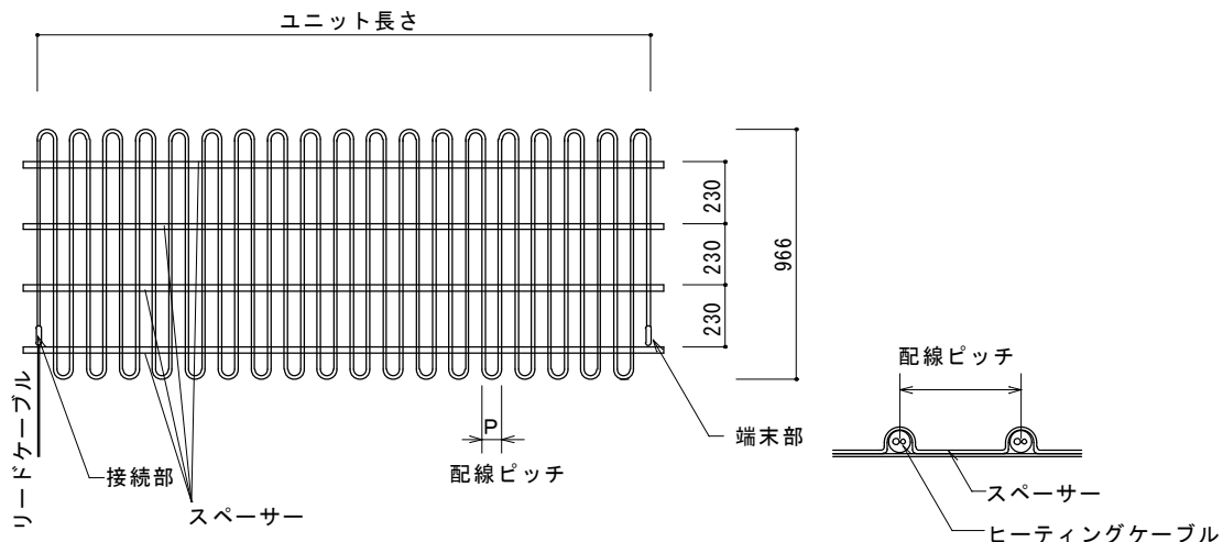
ケーブル断面図 (電磁波対応型)
